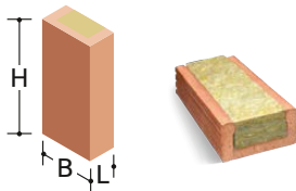
Lücking Anschlagsschale wärmegeämmt
