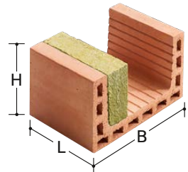
Lücking WU-Schalen wärmegeämmt
