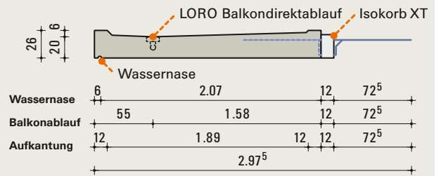
Schnitt B-B
