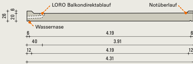
Schnitt A-A
